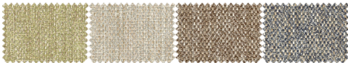
LIBERO_333
