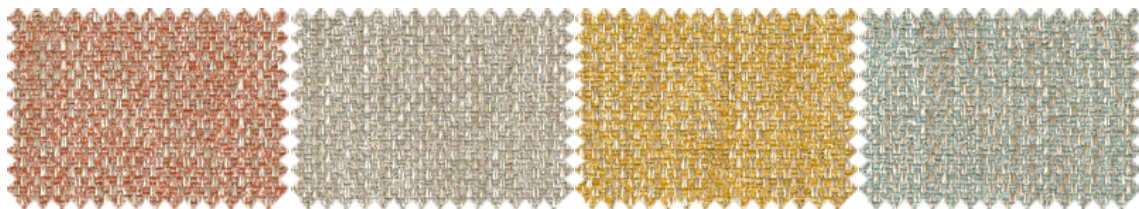
LIBERO_30
