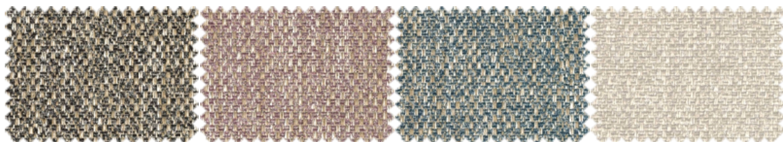
LIBERO_384
